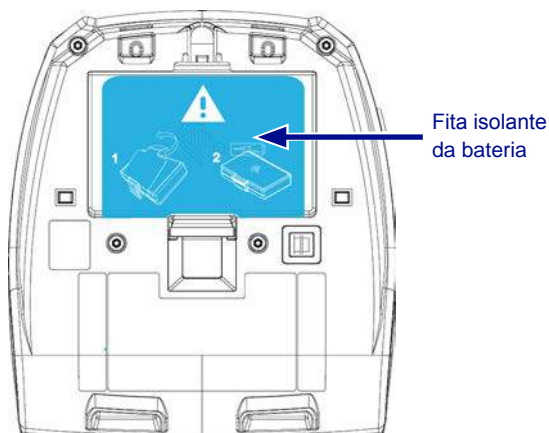
Figura 4 • Remoção da fita isolante da bateria.
