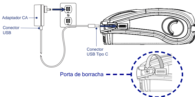
Figura 6 • Adaptador CA-para-USB
