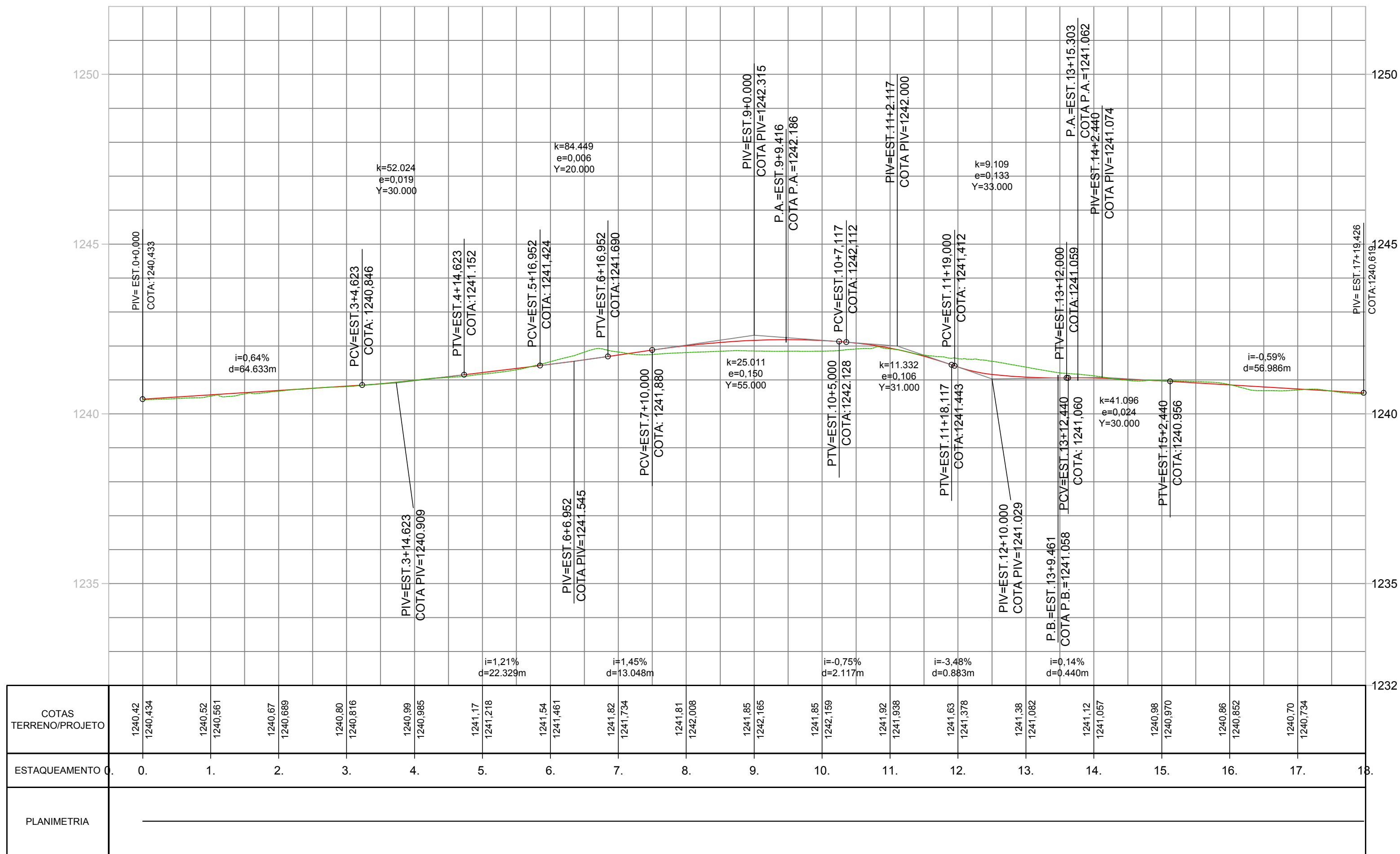
PERFIL V73-OAE(Alça Leste-Oeste)
