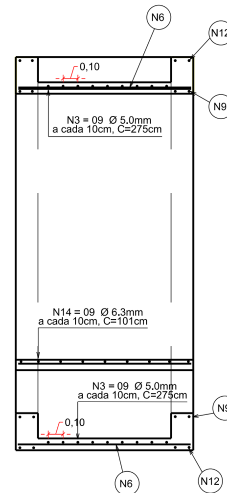
CORTE C-C
