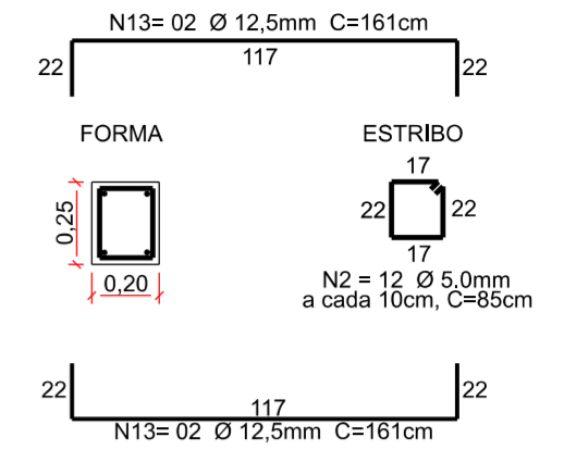
DETALHE2 Esc: 1:25
