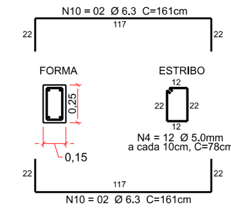
DETALHE1 - (x2)
