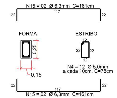
DETALHE1 - (x2) Esc: 1:25
