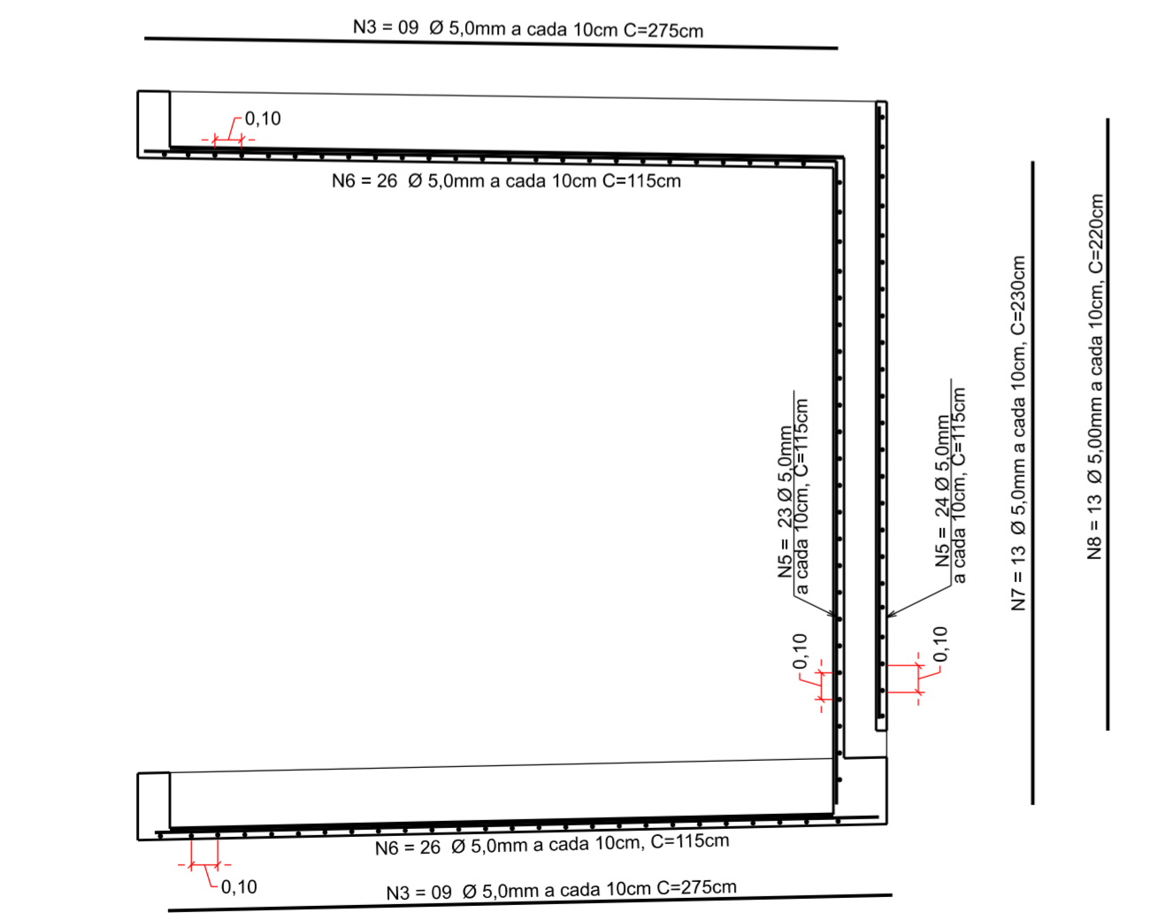
VISTA LATERAL (1º MÓDULO) Esc: 1:25
