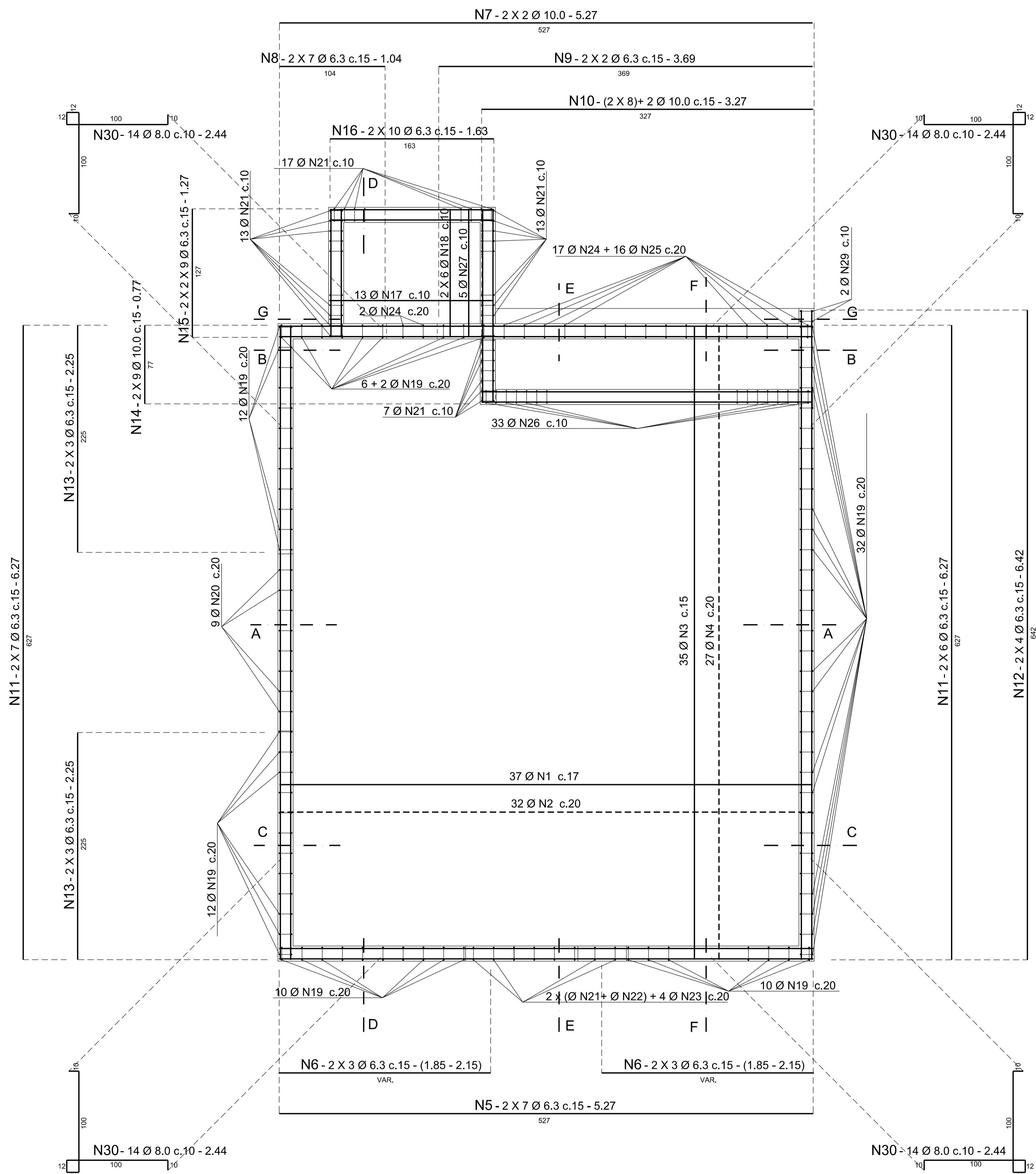
PLANTA BAIXA
