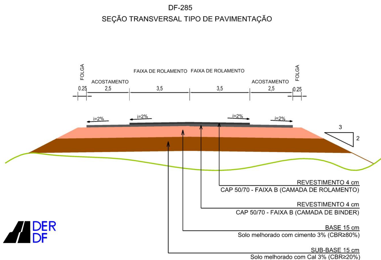
Figura 1 Seção Transversal Tipo da Pavimentação da DF-285
