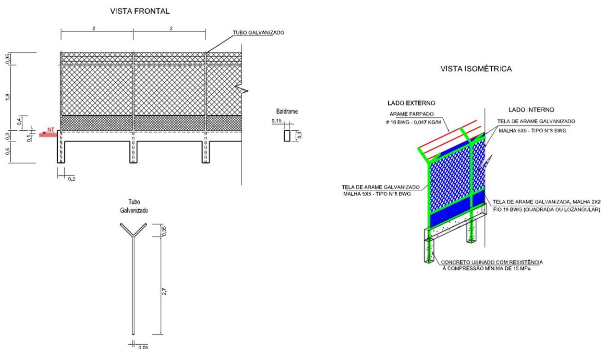
Figura 8 - Modelo de alambrado direcionador de fauna indicado.
