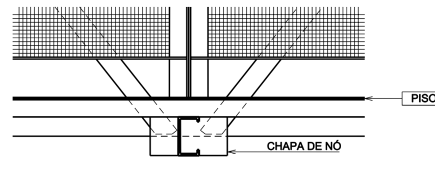
CORTE 1-2
