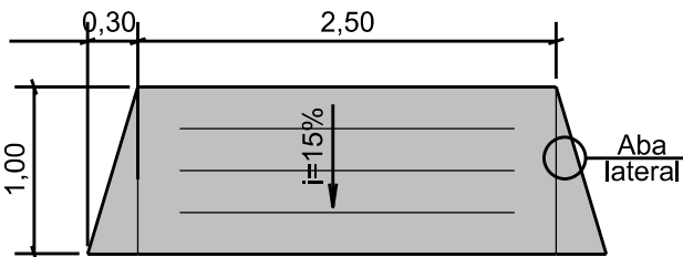
DETALHE 01 - REBAIXAMENTO DE CALÇADA
