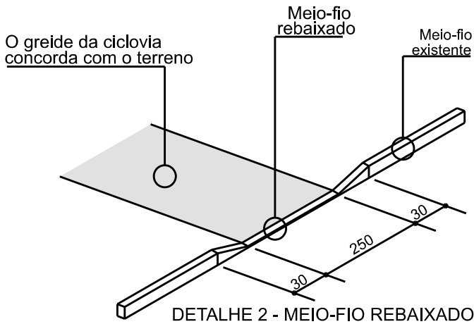
DETALHE 2 - MEIO-FIO REBAIXADO
