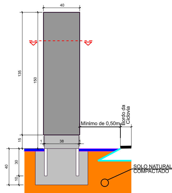
TOTEM - VISTA FRONTAL
