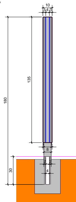
TOTEM - VISTA LATERAL
