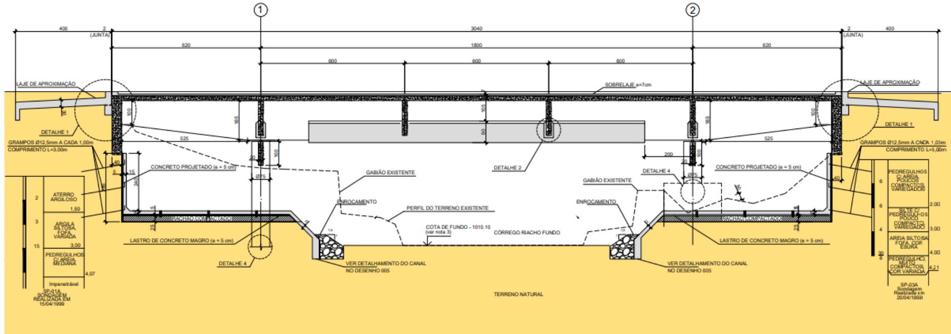
Figura 3: Representação da Seção Transversal com o Alargamento do Canal e Drenagem e Contenção do encabeçamento.
