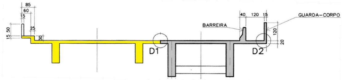
Figura 1: Seção transversal típica da Ponte + Alargamento
