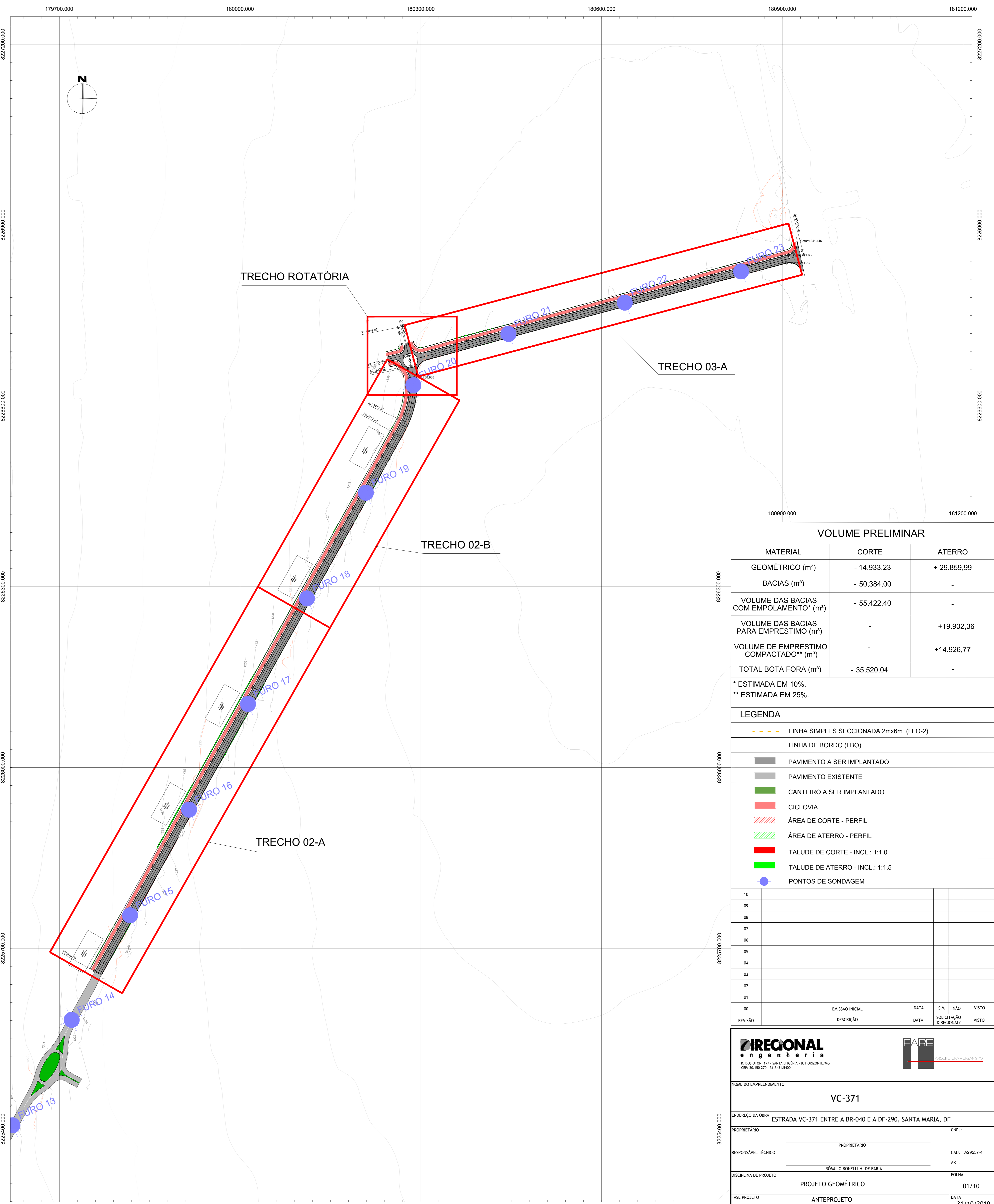
PLANTA GERAL ESC.: 1/2500
