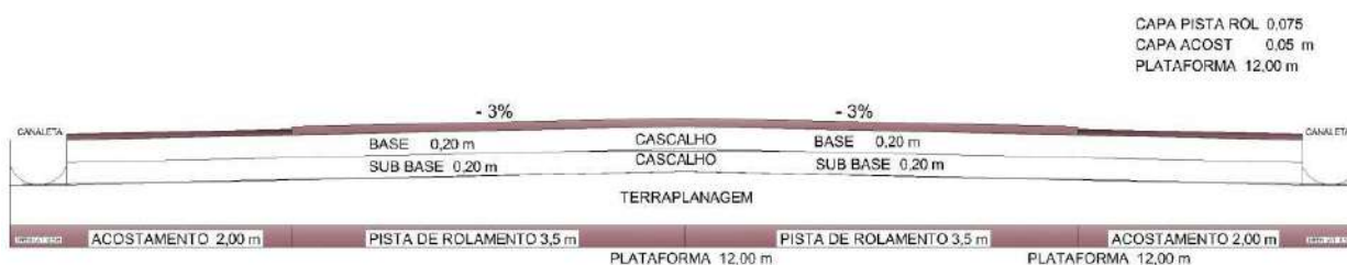
Figura 1 Seção Transversal Tipo da Pavimentação da VC-383 e VC-379
