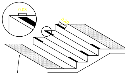
SINALIZAÇÃO VISUAL DE DEGRAUS EM BORRACHA, COR PRETO OU AMARELO, DIM.: 20X3CM COM FIXAÇÃO ATRAVÉS DE CÔLA CONTATO.
