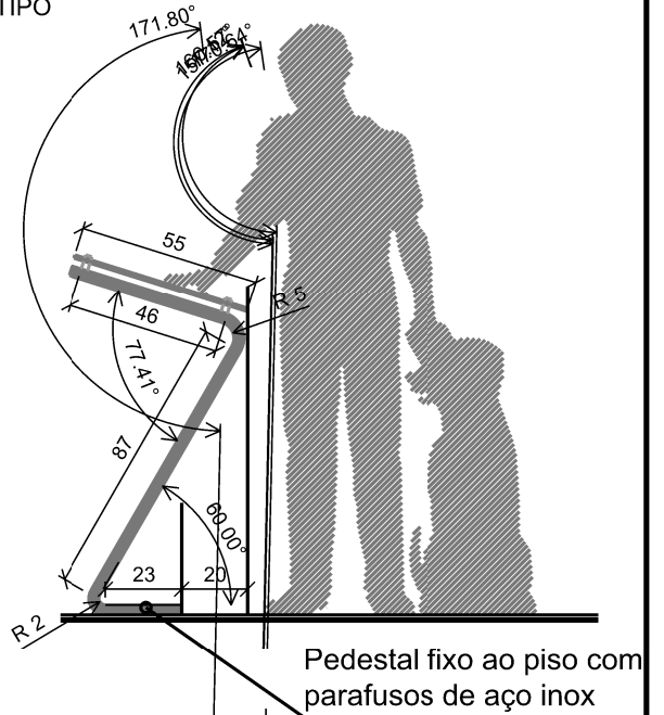
VISTA LATERAL MAPA TÁTIL Esc: 1:25
