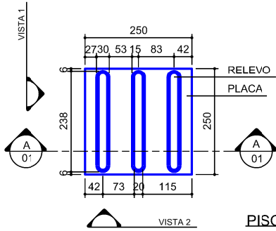
PLANTA BAIXA PISO TÁTIL DIRECIONAL ESC.:1/10
