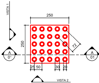
PLANTA BAIXA PISO TÁTIL ALERTA ESC.:1/10
