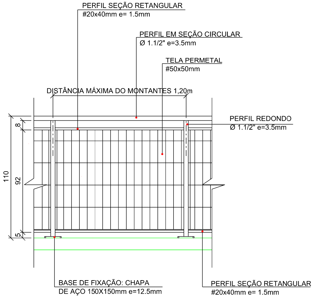
VISTA LATERAL GUARDA CORPO Esc: 1: 20
