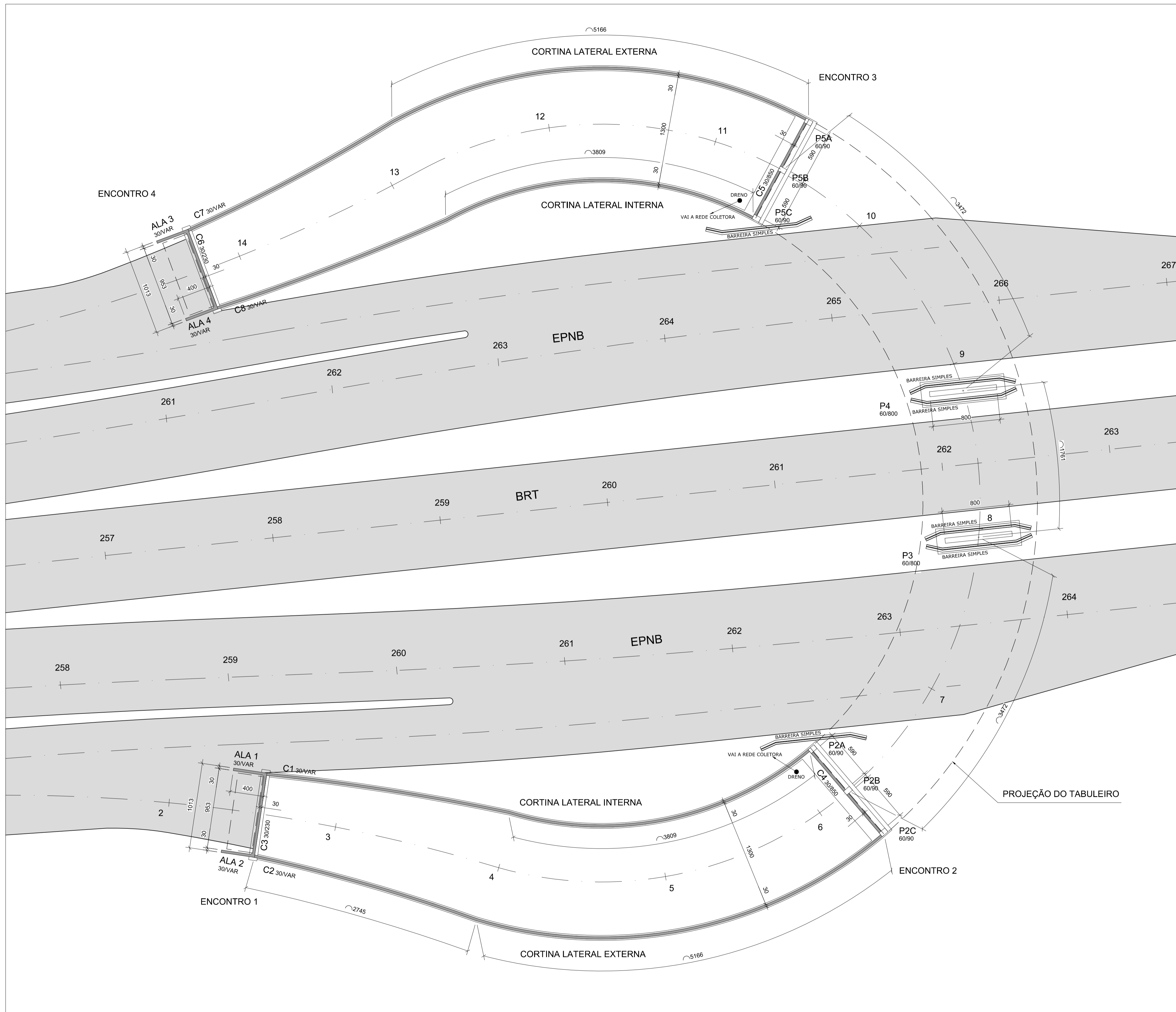
PLANTA DE FORMAS DA MESOESTRUTURA ESC. 1/250
