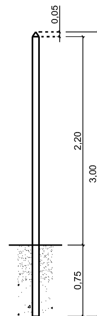
POSTE PARA COLOCAÇÃO DE PLACAS DE SINALIZAÇÃO
