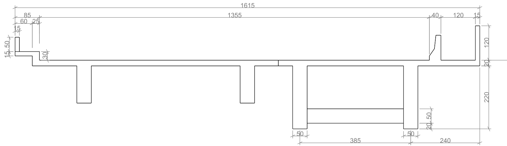
CORTE CD
