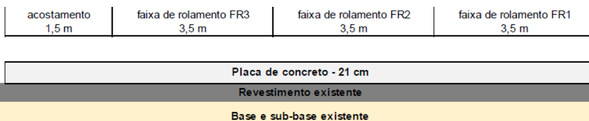
Figura 1 Seção Transversal Tipo / Pavimento Rígido Whitetopping
