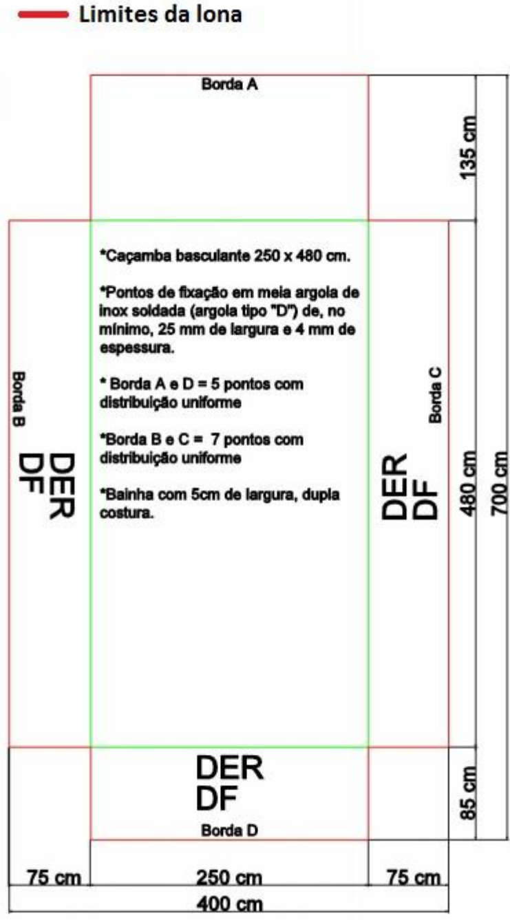
Fig. 01 - Croqui com as dimensões da lona em PEAD. Conforme mostrado, a distribuição dos pontos de fixação, são: na borda A e D - 5 pontos com distâncias uniformes e na borda B e C - 7 pontos com distâncias uniformes.
