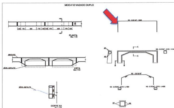
Figura 1 - Projeto Meio fio vazado
