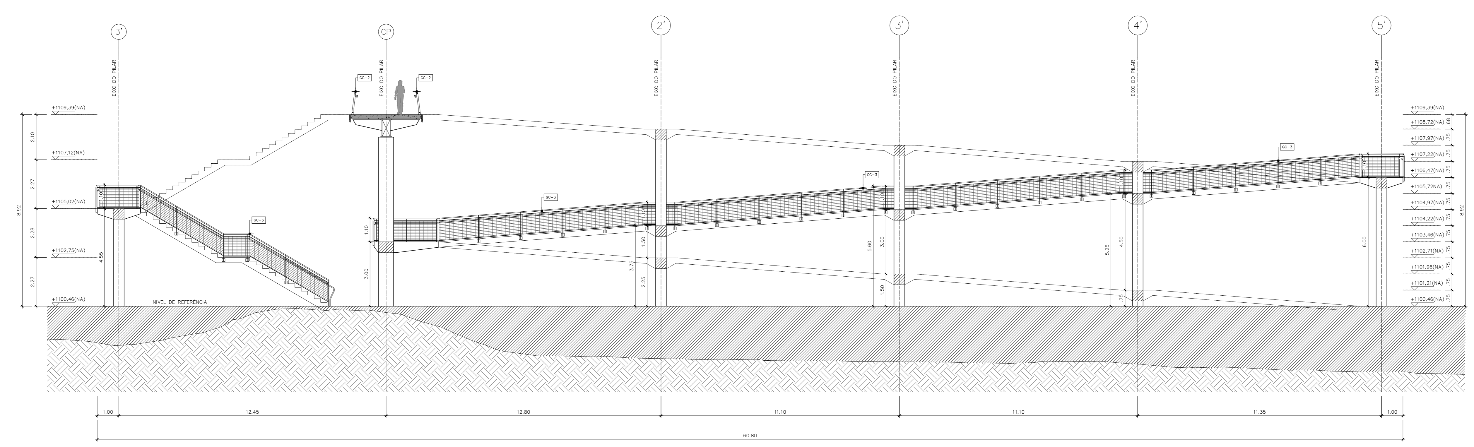
SEÇÃO C PERFIL LONGITUDINAL ESC: 1:100
