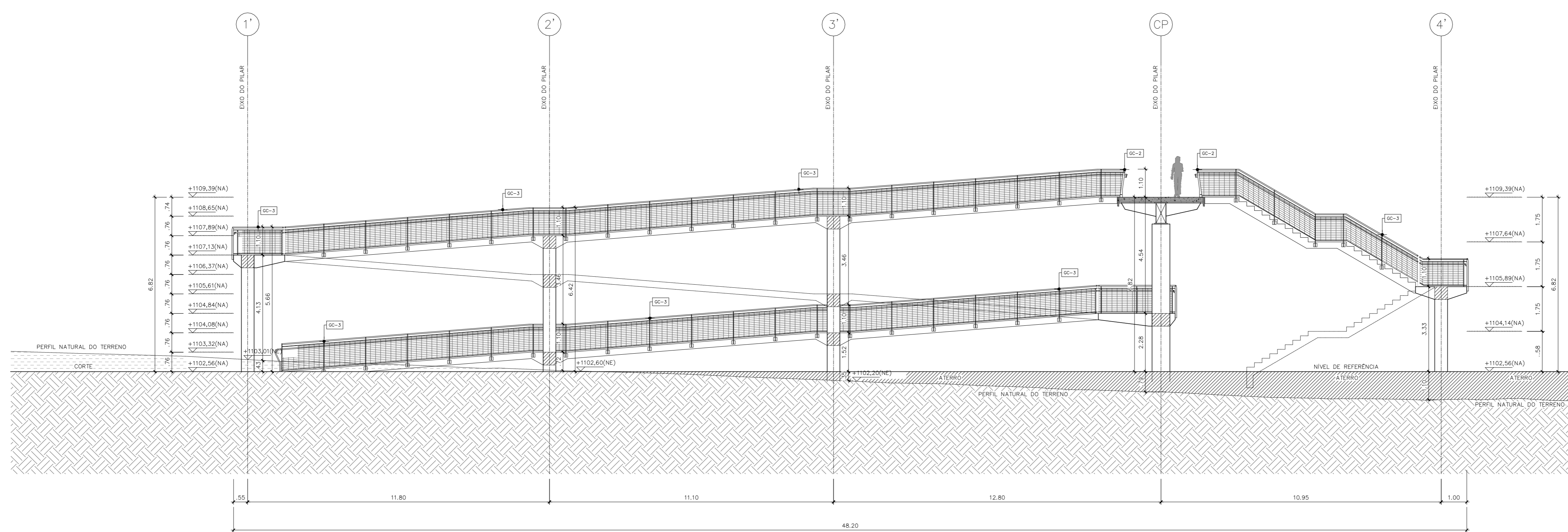
SEÇÃO B PERFIL LONGITUDINAL ESC: 1:100
