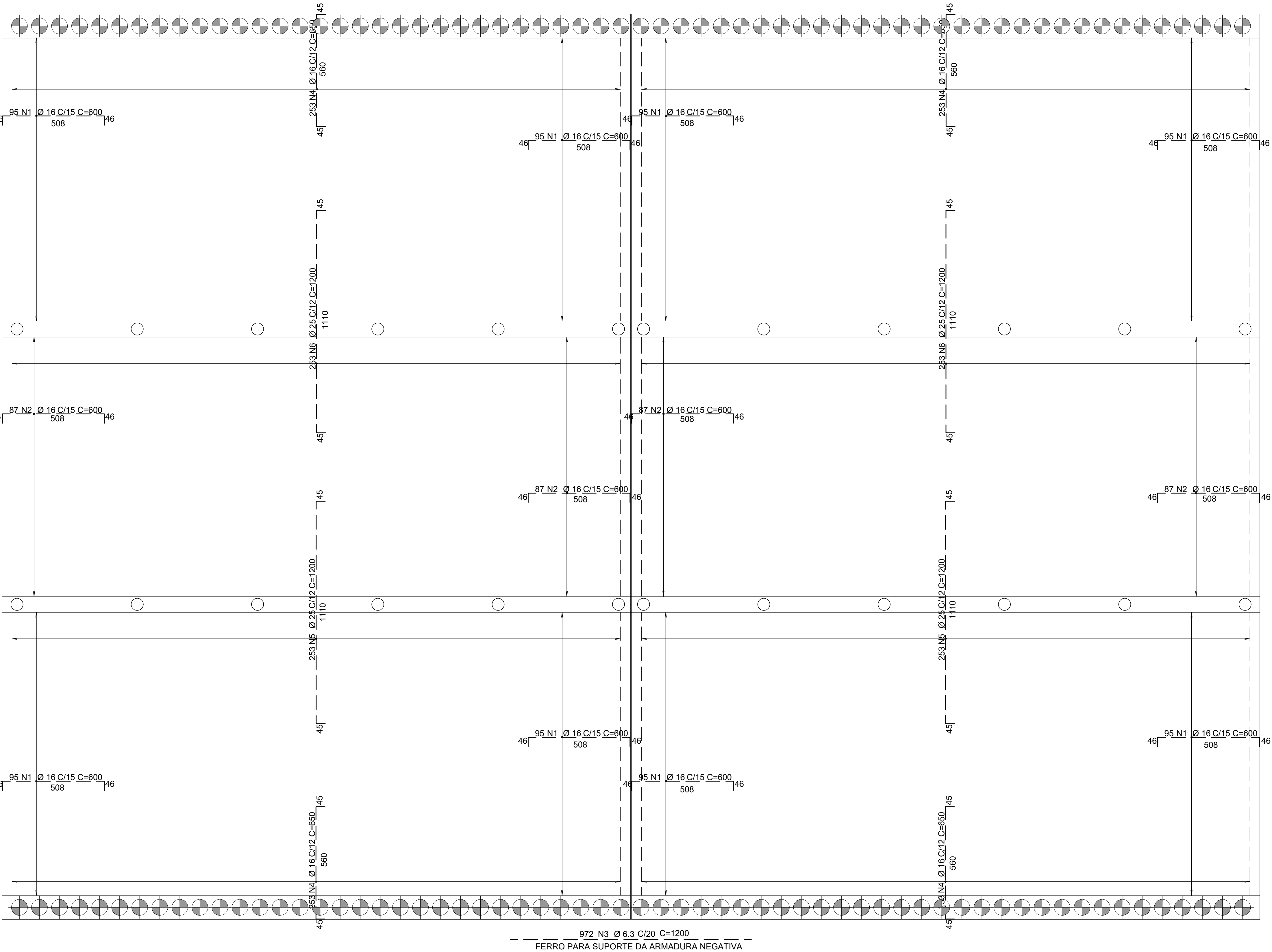
ARM. NEGATIVA DO TABULEIRO ESCALA 1:100
