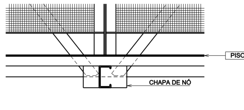
CORTE 1-2
