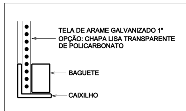
PORMENOR 1 S/ESCALA
