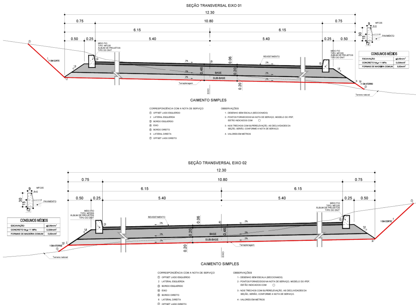
Figura 2 – Seções típicas os Eixos 01 e 02 (Fonte: Projeto de Terraaplenagem - STE Serviços Técnicos e de Engenharia S.A)
