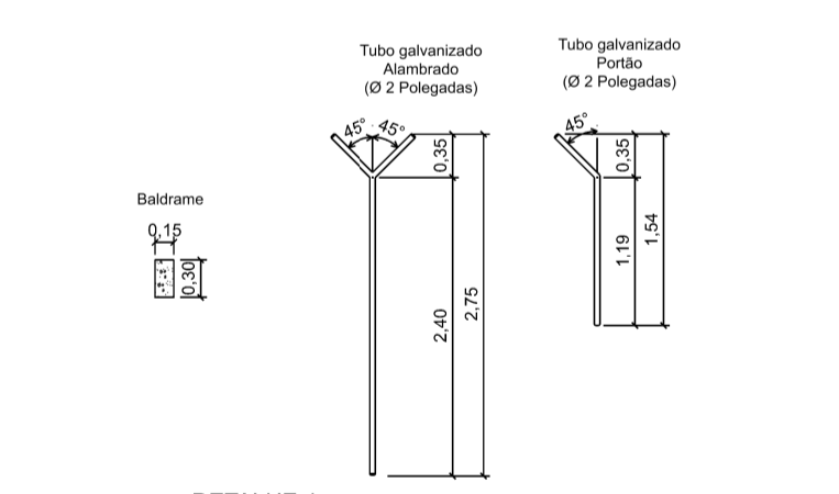
DETALHE 4 BALDRAMES E TUBOS GALVANIZADOS Sem escala
