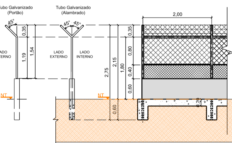
DETALHE 5 CORTE ESQUEMÁTICO DOS TUBOS GALVANIZADOS Sem escala
