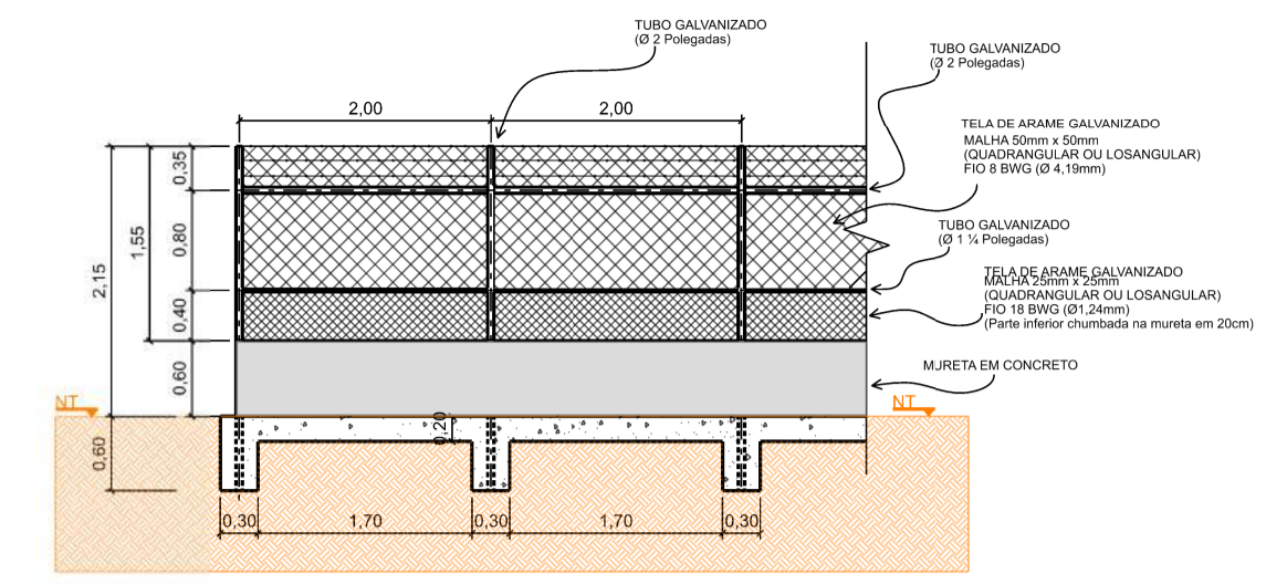
DETALHE 1 CORTE ESQUEMÁTICO DO ALAMBRADO DIRECIONADOR DE FAUNA COM MURETA EM CONCRETO Sem escala
