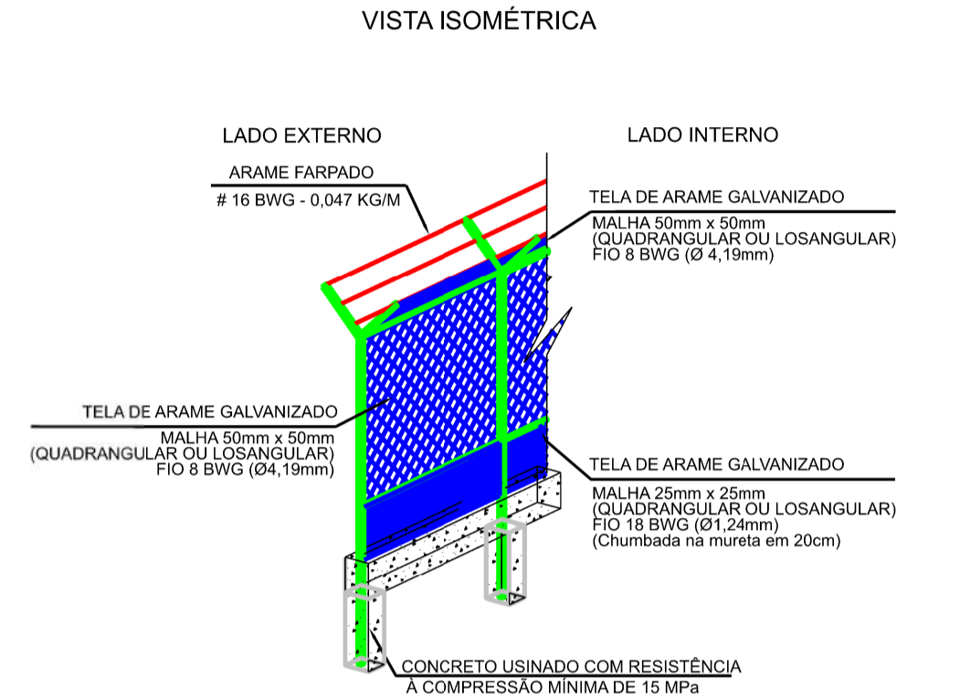
DETALHE 2 ALAMBRADO DIRECIONADOR DE FAUNA COM MURETA EM CONCRETO Vista isométrica - Sem escala
