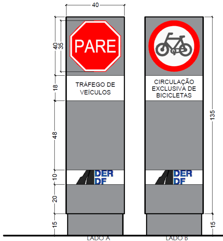
DETALHE TOTEM 01 - R1 Parada obrigatória e R34 Circulação exclusiva de bicicletas
