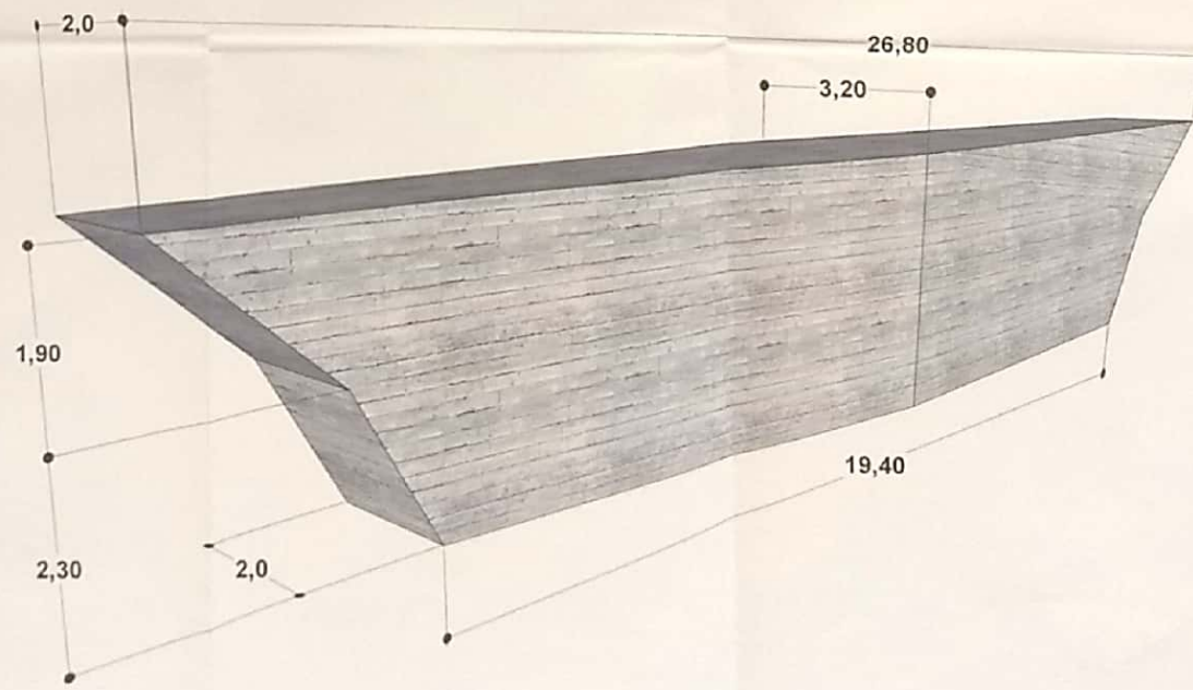
COTAS GERAIS ESC: SEM ESCALA
