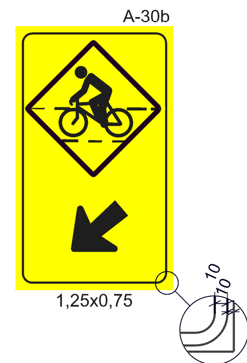
DETALHE PLACA SEM ESCALA
