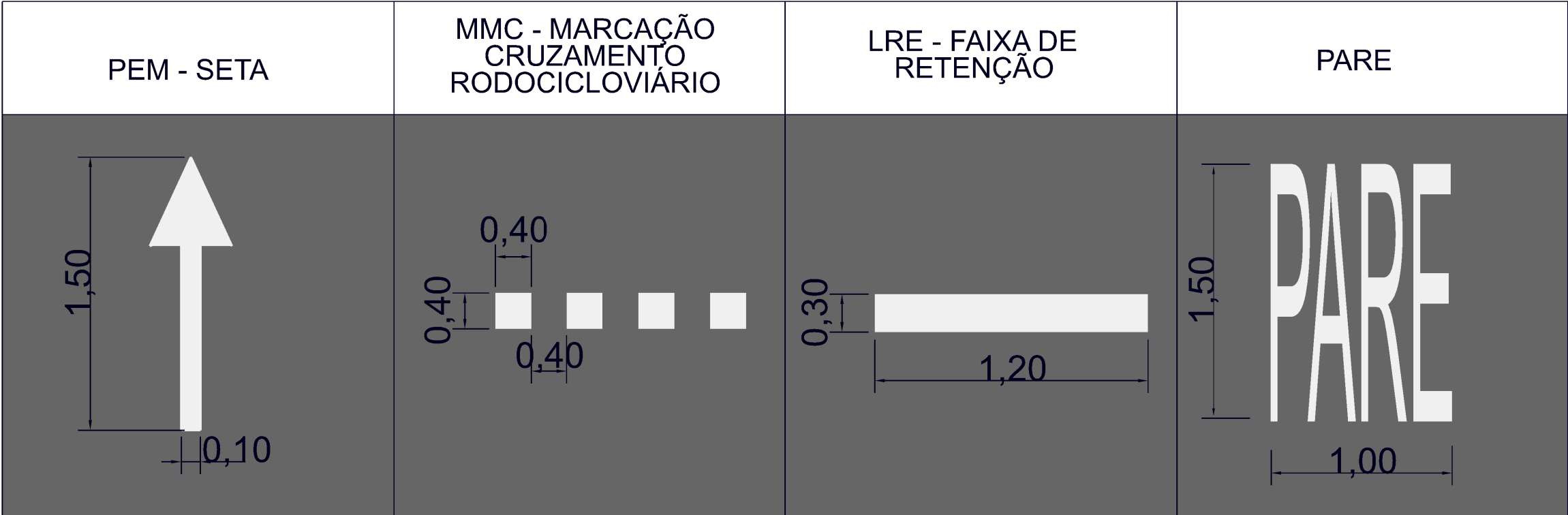
INSCRIÇÃO NO PAVIMENTO - CICLOVIA
