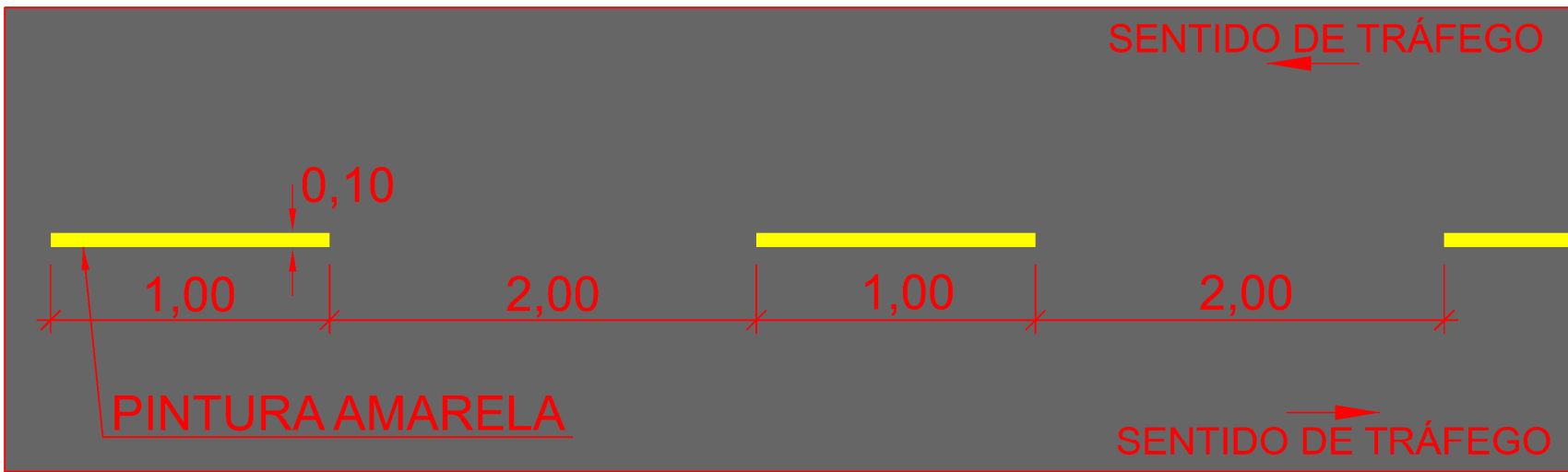
FAIXA SECCIONADA CICLOVIA
