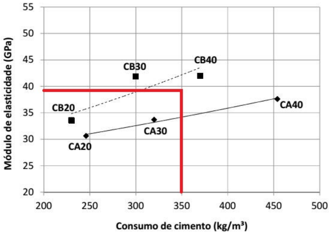
Figura 2 – Módulo de elasticidade em função do consumo de cimento.
