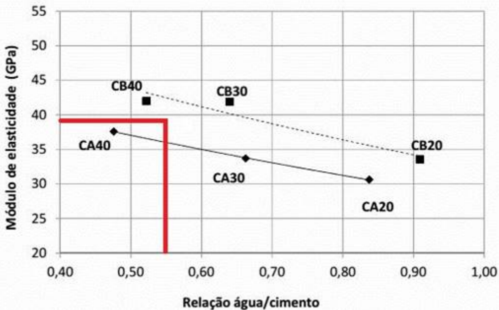
Figura 3 – Módulo de elasticidade em função da relação água/cimento
