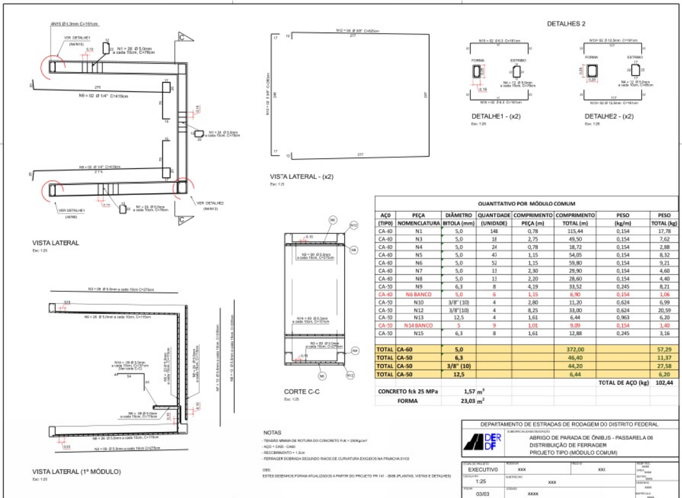
Fig. 02 - Imagem da distribuição das barras.
