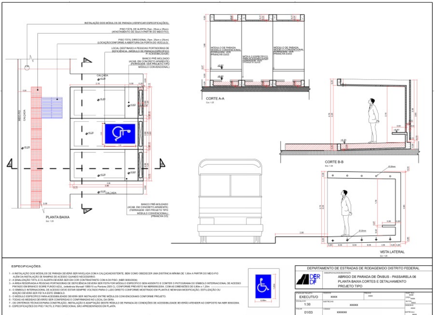
Fig. 01 - Imagem com as dimensões da parada de ônibus;
