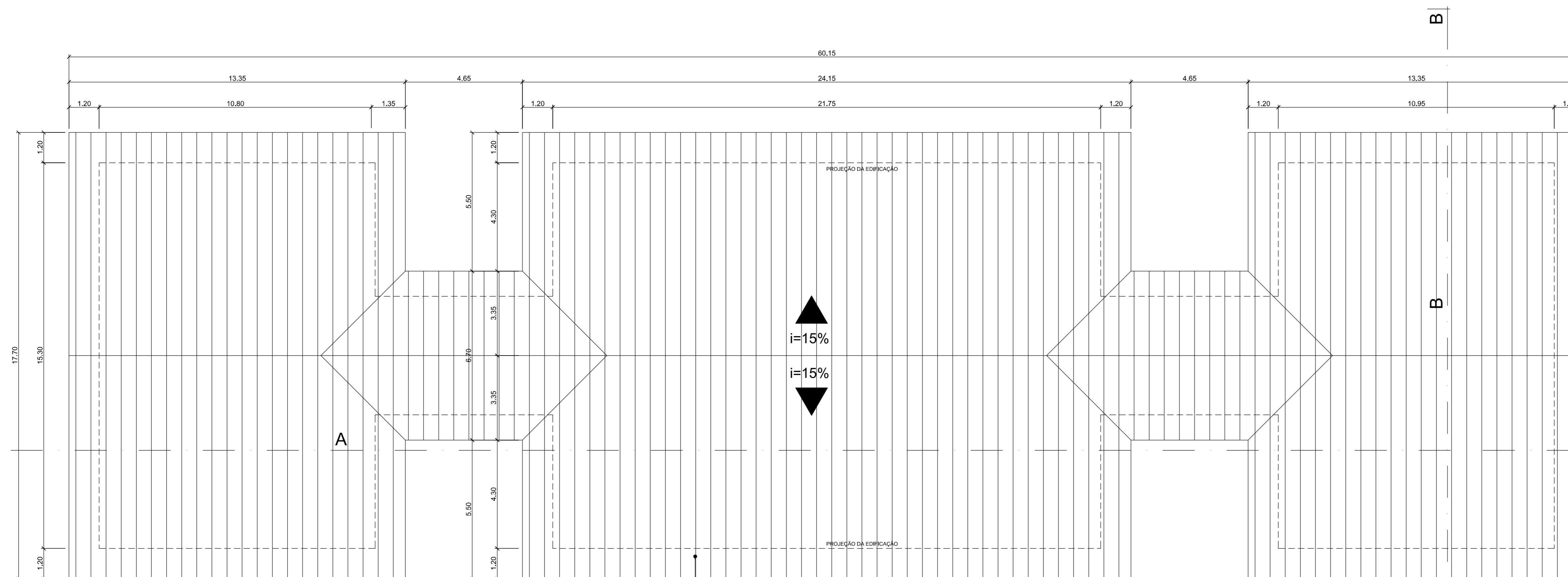
PLANTA COBERTURA ESC 1:100
