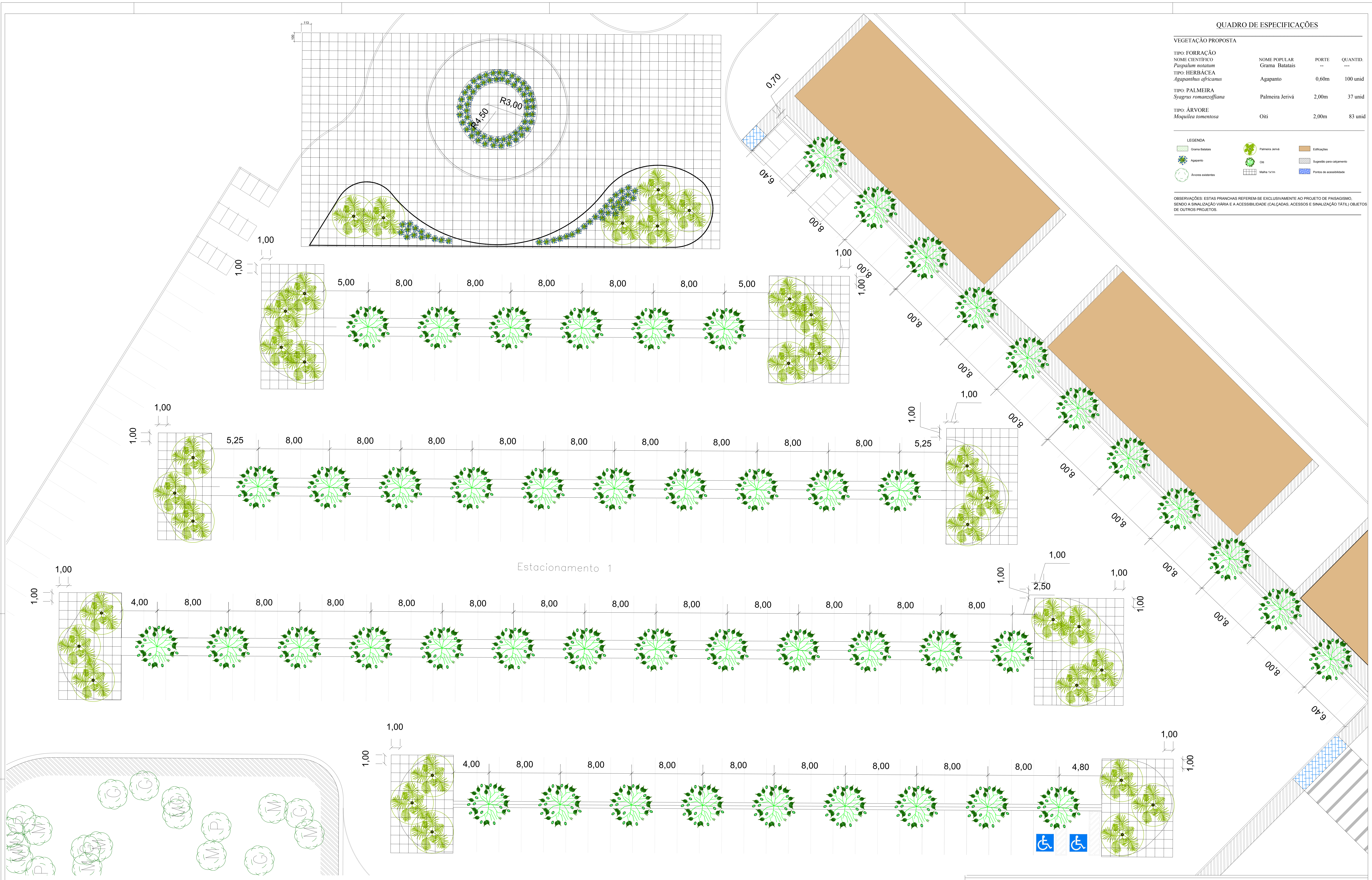
DETALHE - ESTACIONAMENTO 1 escala 1:125
